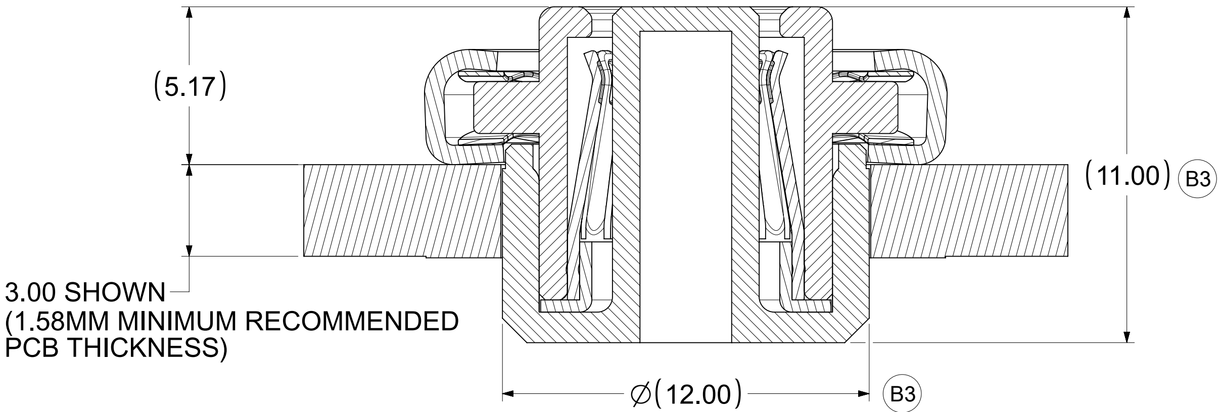
SECTION A-A
