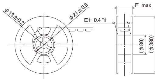
■ Reel Diagram
