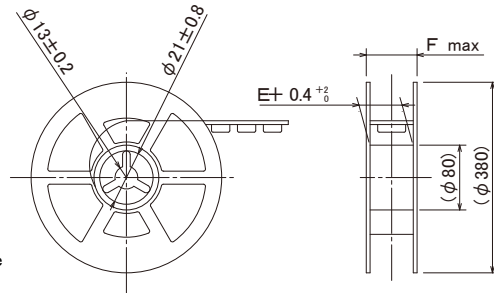
■ Reel Diagram
