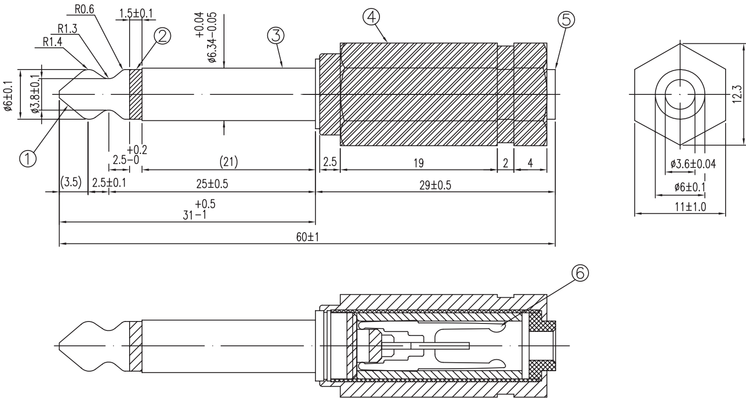
Ø6.3 Mono Plug
