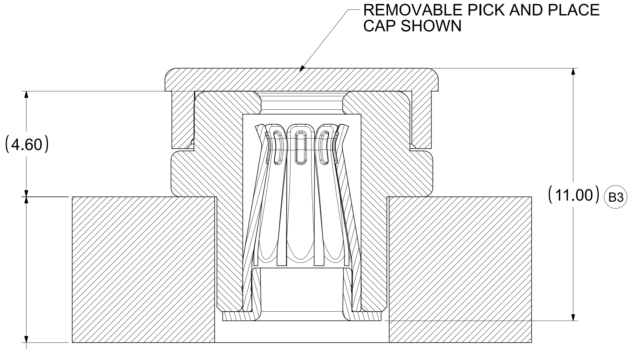
SECTION A-A
