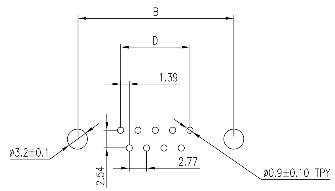
P.C.B LAYOUT
