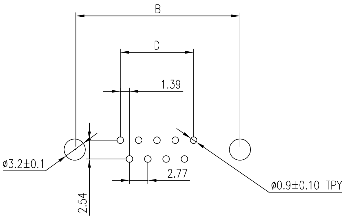
P.C.B LAYOUT
