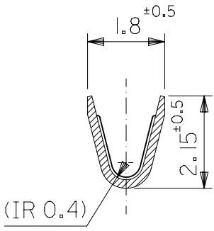
断面 B-B SECT.B-B
