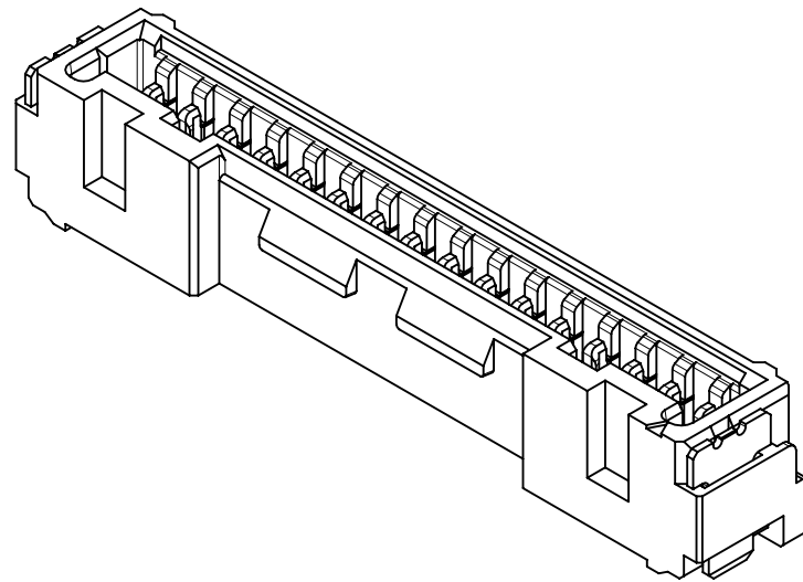
15-16 極 15-16 CIRCUIT
