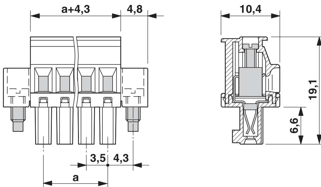
尺寸图
