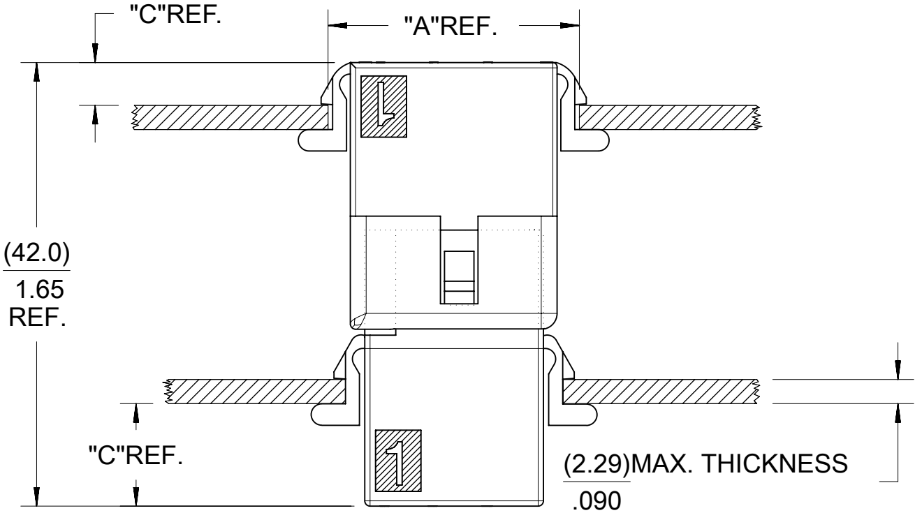
RECEPTACLE 1292-R
