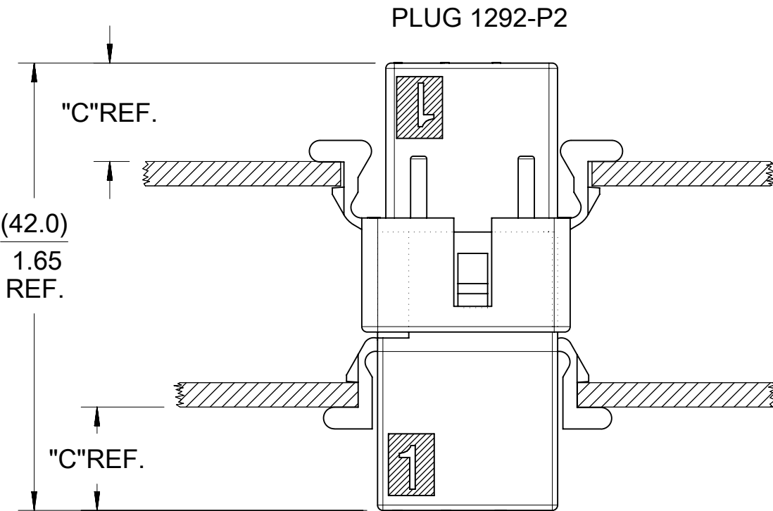
RECEPTACLE 1292-R
