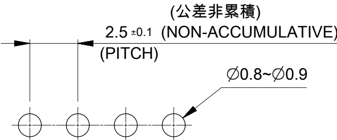
基板取付穴推奨寸法 RECOMMENDED PCB HOLE DIMENSION (t=1.6)
