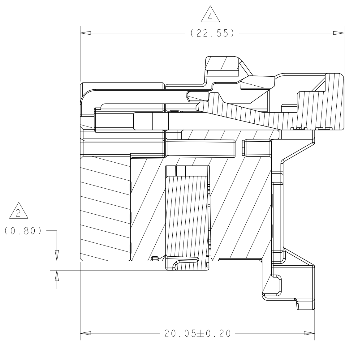
SECTION D-D
