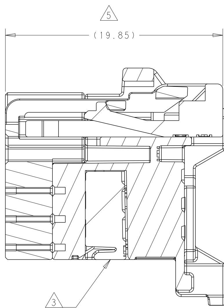
SECTION D-D
