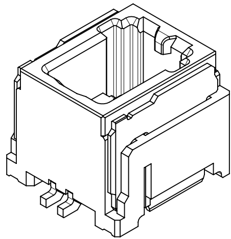
4-6極 4-6 CIRCUIT
